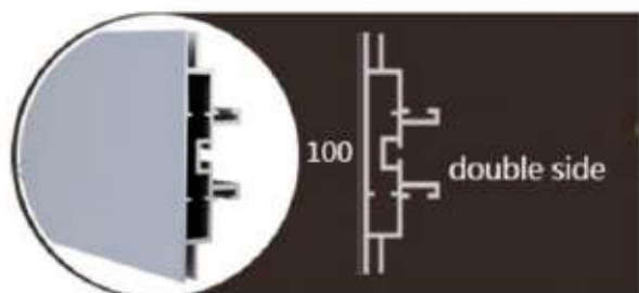
PERFIL FRAMELESS DE 10CM PROFUNDIDAD Formato de venta perfil 3mts.
