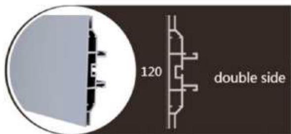
PERFIL FRAMELESS DE 12CM PROFUNDIDAD Formato de venta perfil 3mts.
